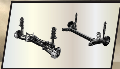
ប្រព័ន្ធដើងក្រោមផ្តល់ធានាសុវត្ថិភាព និងកាត់បន្ថយលោត
